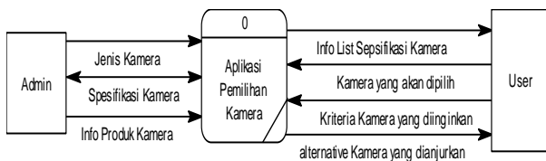
Gambar 1. Diagram Konteks Aplikasi Pemilihan Kamera Dengan Adaptive Software Development Dan Weighted Product
